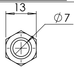
M8 NUT
