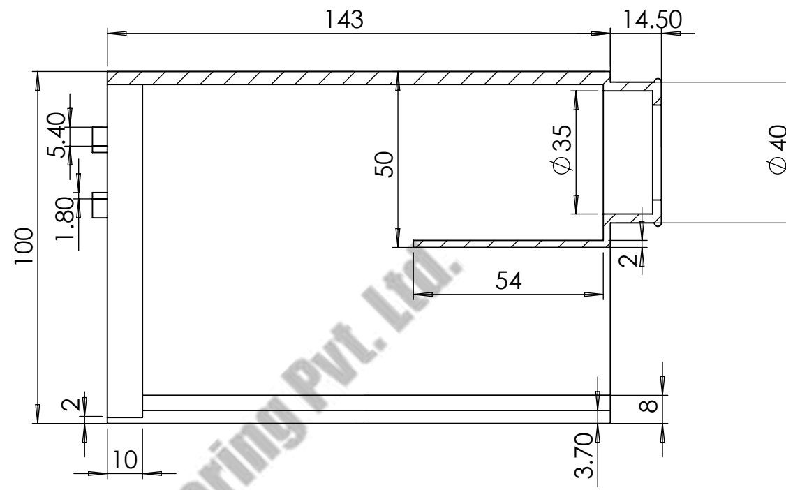
SECTION A-A SCALE 1 : 1.5
