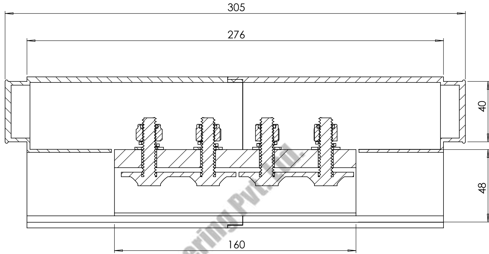
SECTION A-A SCALE 1 : 1.5
